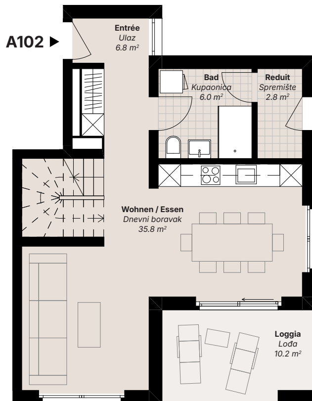
Erdgeschoss Prizemlje
